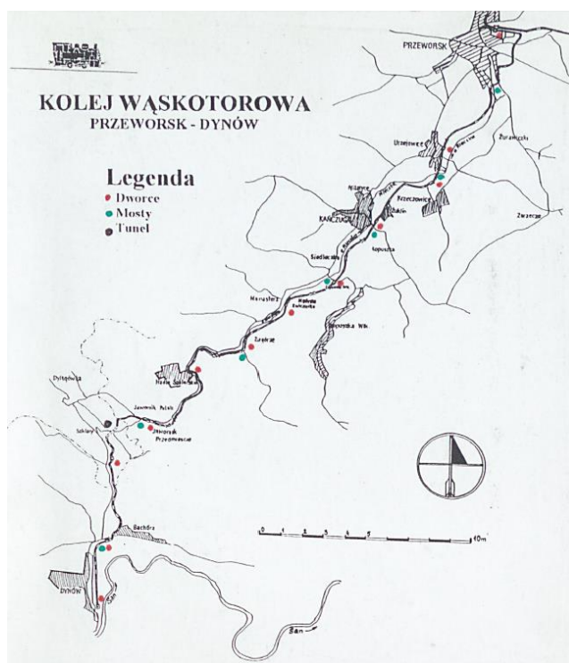
Fot. 20. Plan kolejki wąskotorowej Przeworsk-Dynów.
